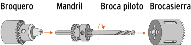
Ensamble
